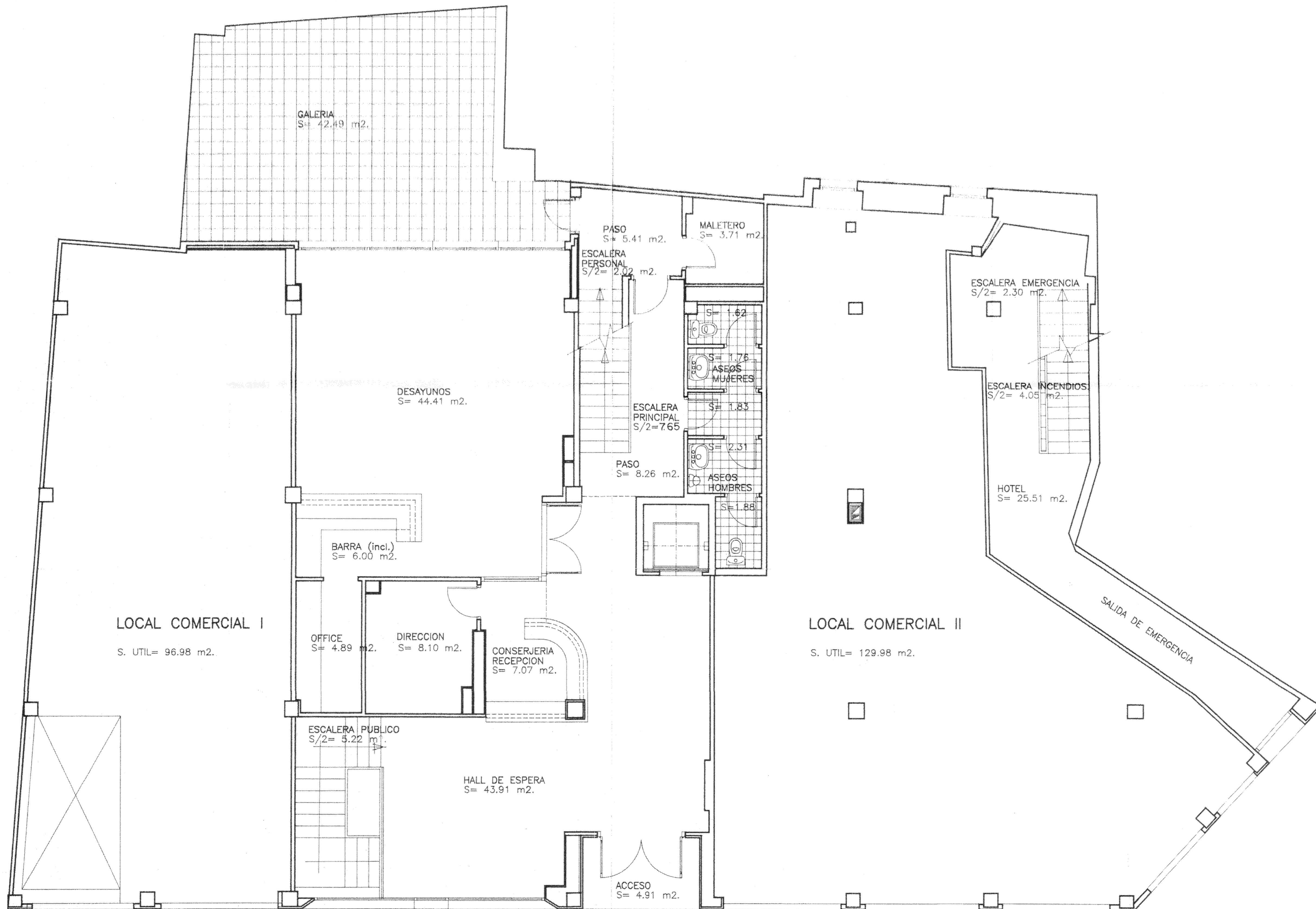
planta baja. escala 1:50.
